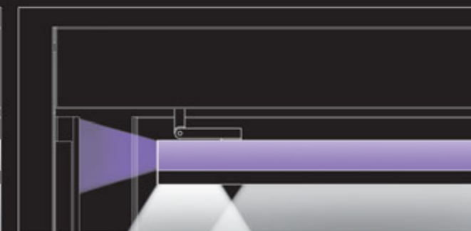
LD5X-LED-RGB Esquema de funcionamento iluminação directa-indirecta Luz LED branca neutra / Cor a pedido Ascensores Color Glas® / Corte vertical
